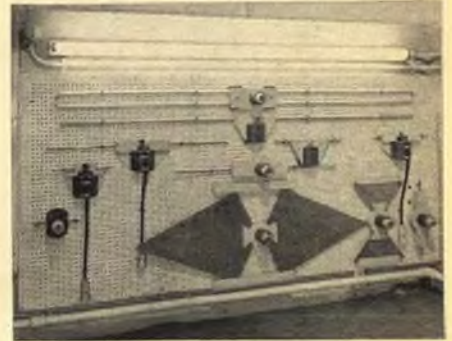
Bild 6 ▶ Zusammenstellung der Meß- und Eichantennen
