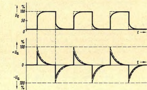
Bild 4.9. RC-Differenzglied; Einfluß des Innenwiderstandes im Pulsspannungserzeuger auf den zeitlichen Verlauf der Größen U_e und U_a
