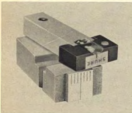
Bild 3. Der Skatingkraft-Detektor
