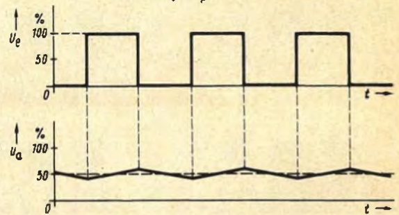
Bild 4.6. RC-Integrierglied; \tau = 5 \cdot t_i \tau = 5 \cdot t_p
