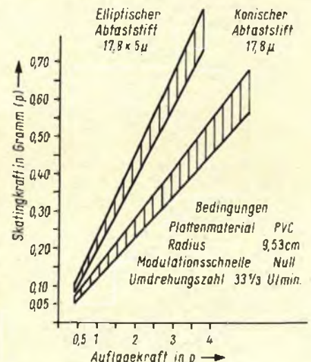
Bild 5. Skatingkraft in Abhängigkeit von der Auflagekraft
