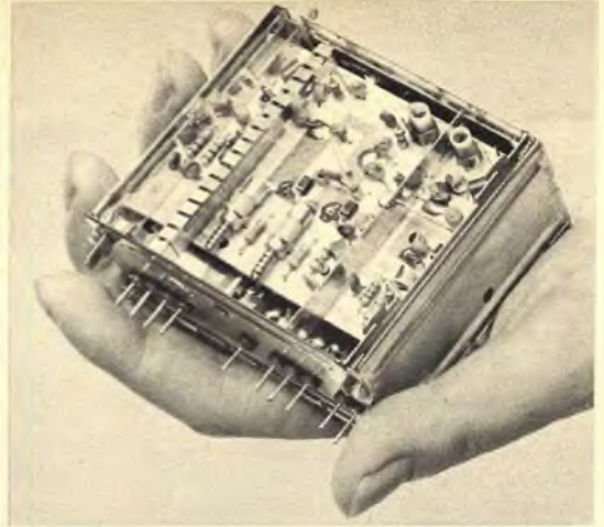
Bild 3 ▶ Vartuner Typ 162 mit geöffneter UHF-Seite. Der Größen- vergleich mit der Hand zeigt die geringen Abmessun- gen dieses von AEG- Telefunken entwickel- ten Tuners
