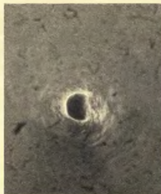
Bild 11. Einseitig abgeschliffener Diamantabtaststift nach Lebensdauerprüfung ohne Kompensation der Skatingkraft
