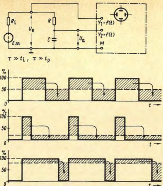
Bild 4.8. RC-Integrierglied; Ausgangsgleichspannung in Abhängigkeit vom Tastverhältnis der Impulsfolge am Eingang
