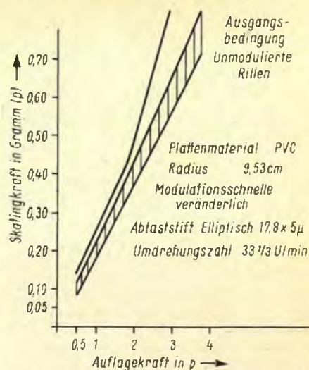
Bild 7. Typische Auswirkungen der Skatingkraft in Abhängigkeit von der Auflagekraft (modulierte Rillen und elliptischer Abtaststift)
