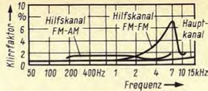
Bild 3. Klirrfaktor-Frequenzgang des FM-FM- und des FM-AM-SSB-Multiplex-Verfahrens für den Haupt- und den Hilfskanal
