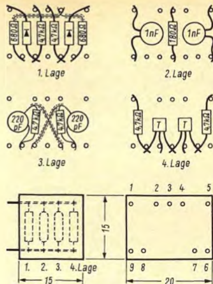
Bild 3. So werden die Bauelemente lagenweise geschichtet
