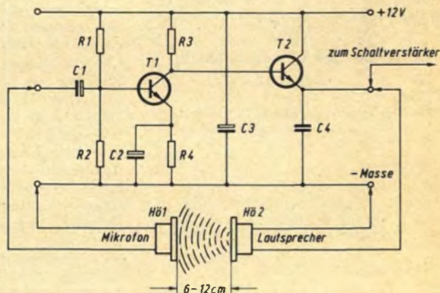
Bild 1. Schaltung einer einfachen akustischen Schranke mit einer Reichweite von etwa 12...50 cm
