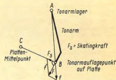
Bild 1. Entstehung der Skatingkraft mit Kräfteparallelogramm
