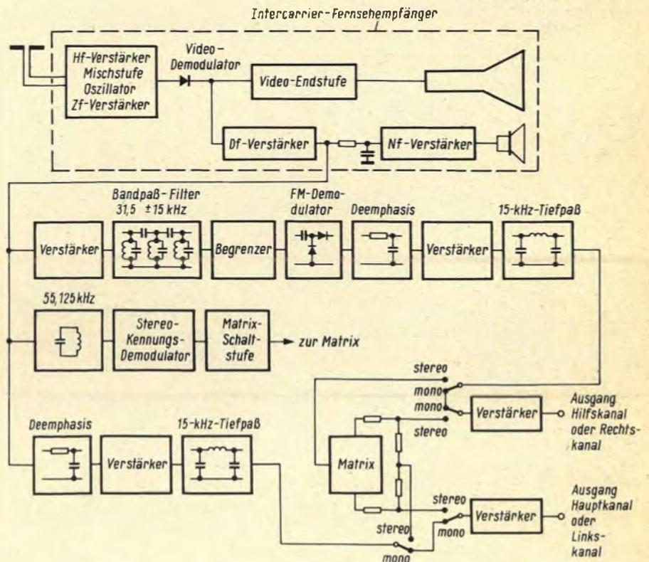
Bild 9. Anschlußschema und grundsätzlicher Aufbau eines Empfangsadaptors nach dem FM-FM-System zum Nachrüsten eines Intercarriempfängers
